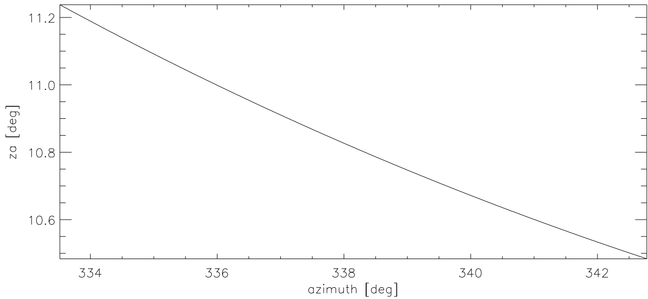
za vs az
