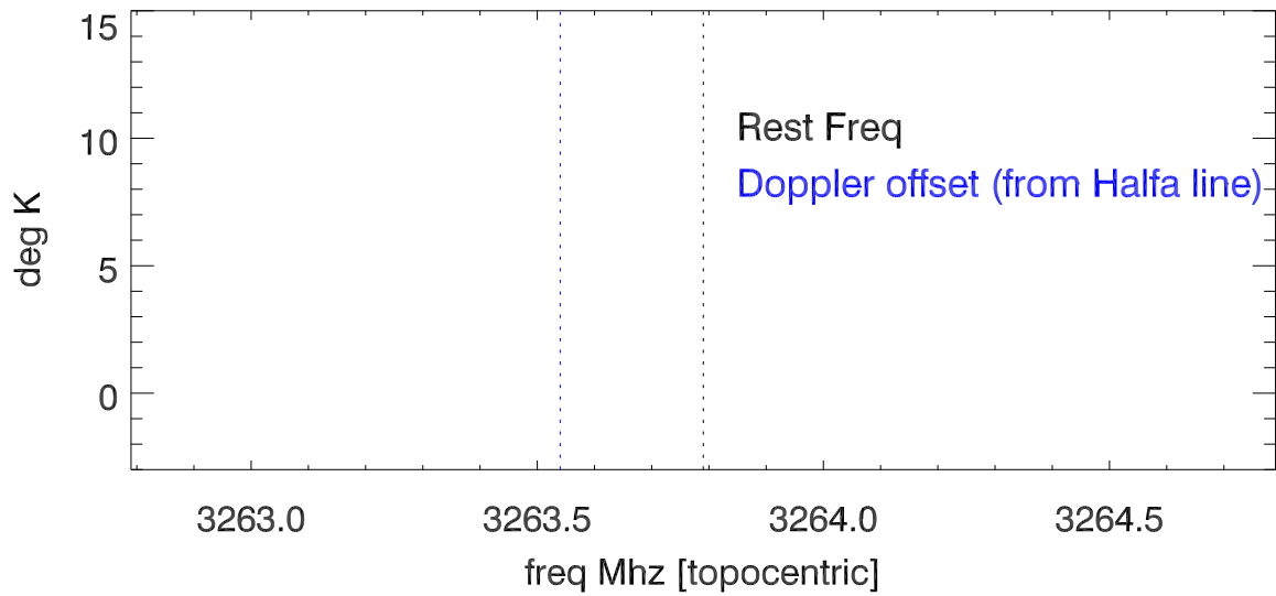
02jun10 a2463 SBH CH lines: 3263.79 Mhz
