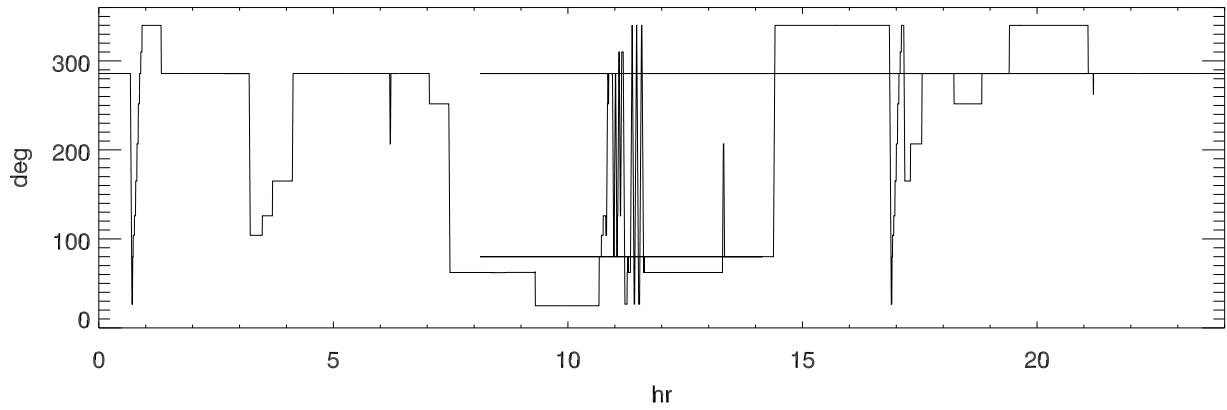
151105 turret Actual position
