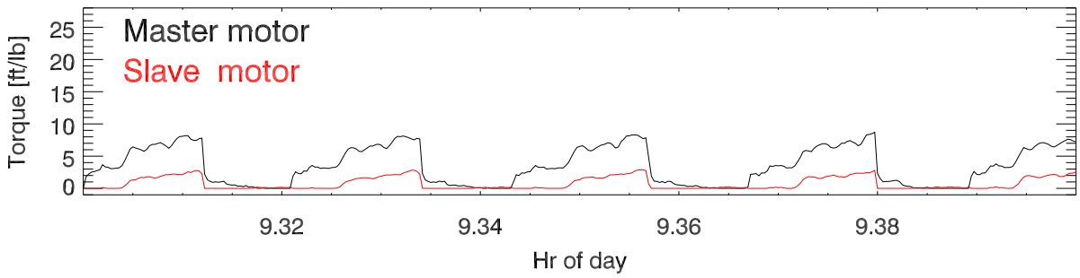
Motor torques
