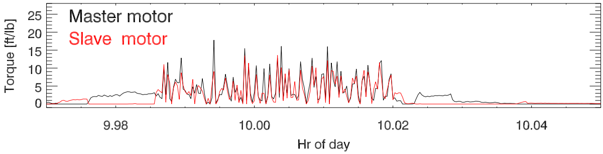
Motor torques
