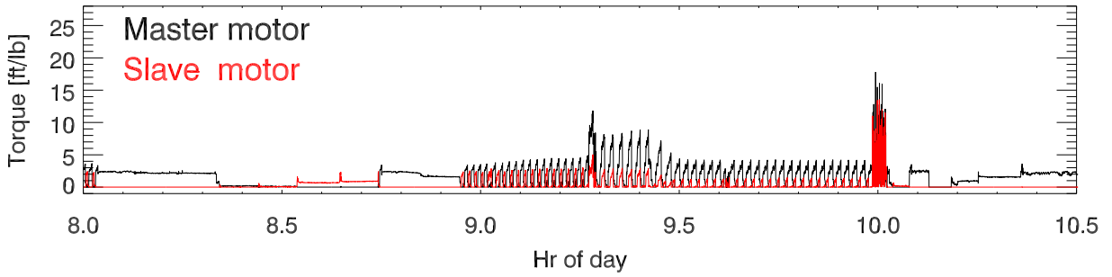
Motor torques
