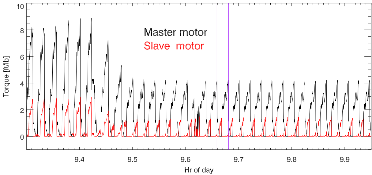
Motor torques
