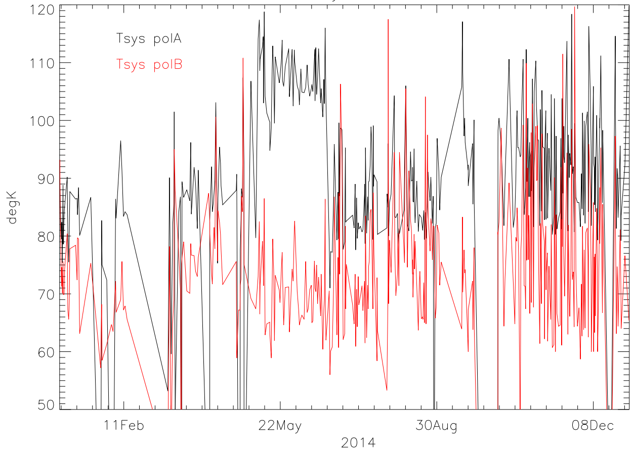
430ch TsysA-TsysB 2014
