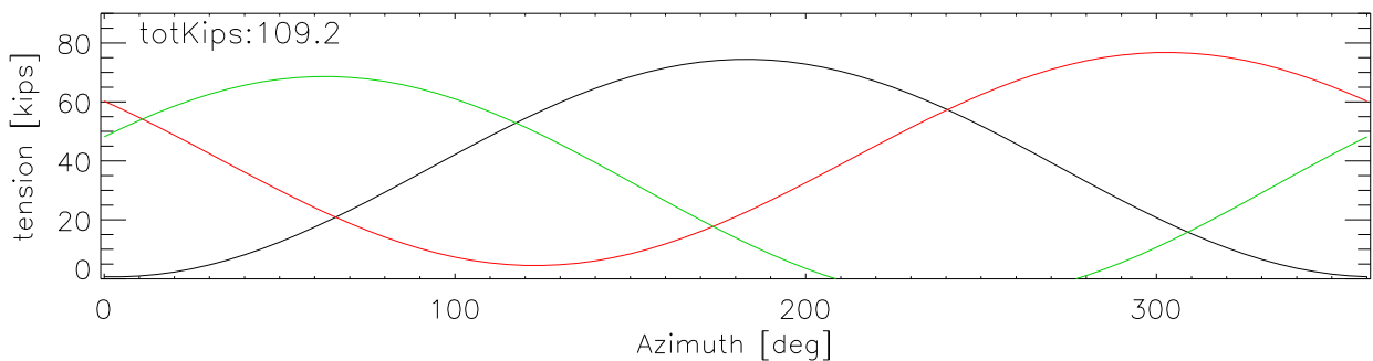
dome za=19.7
