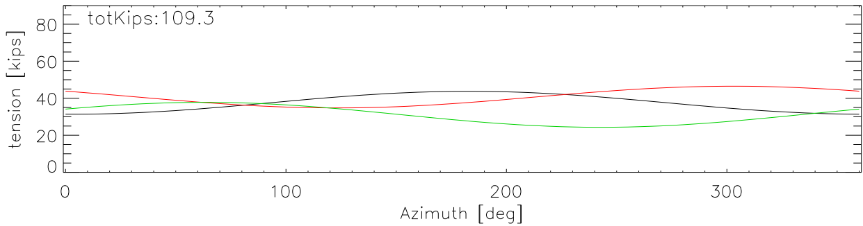
dome za=15.0
