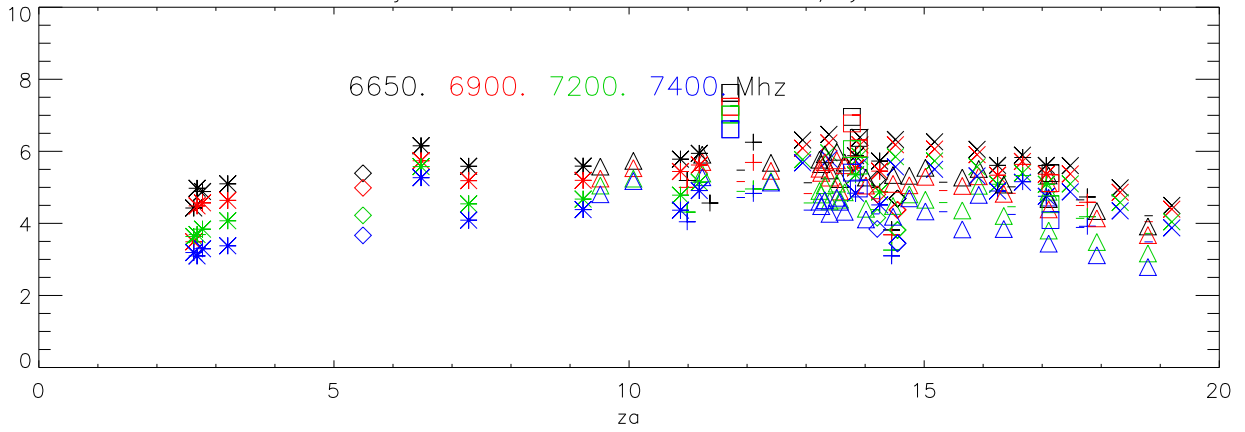
T_{\text{sys}}
