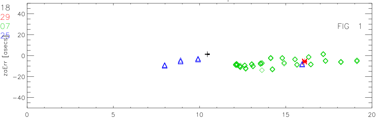
01mar15 to 31mar15 lbw 116 pnts. za error vs za
