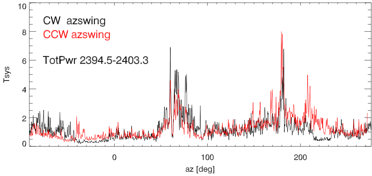
12oct11 sbw power vs az at 2400Mhz. polA
