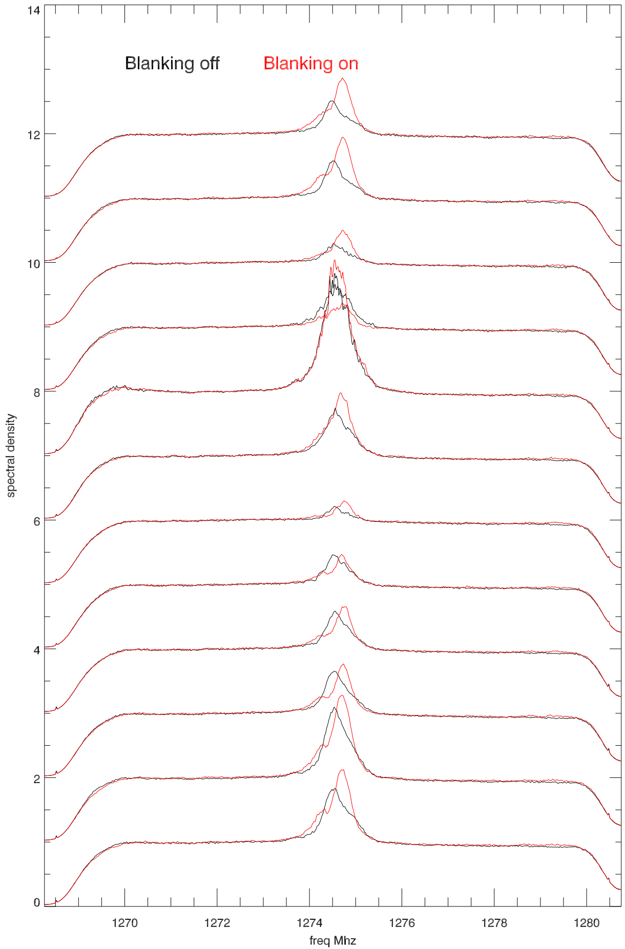
29apr13 puntaBorinquen radar 12 1 sec spectra
