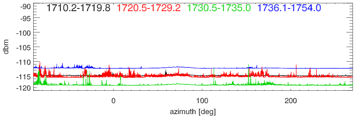
TotPwr 1710-1750
