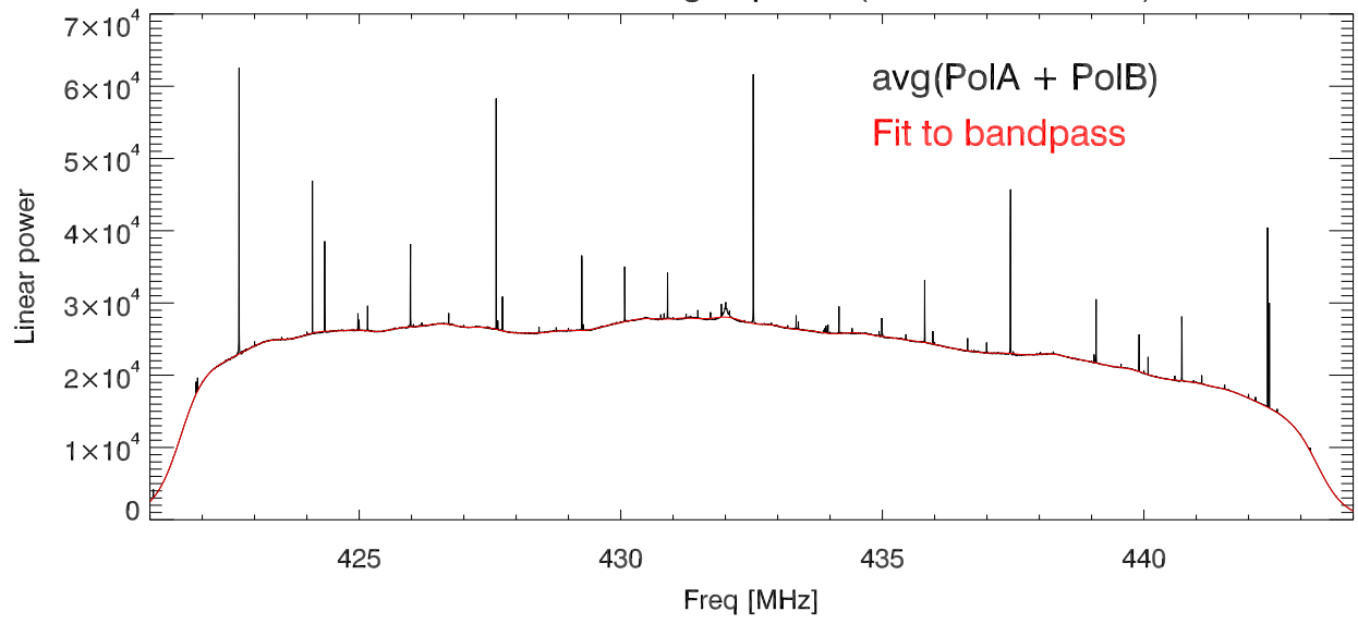
(avgSpectra / fitToBandpass) - 1.
