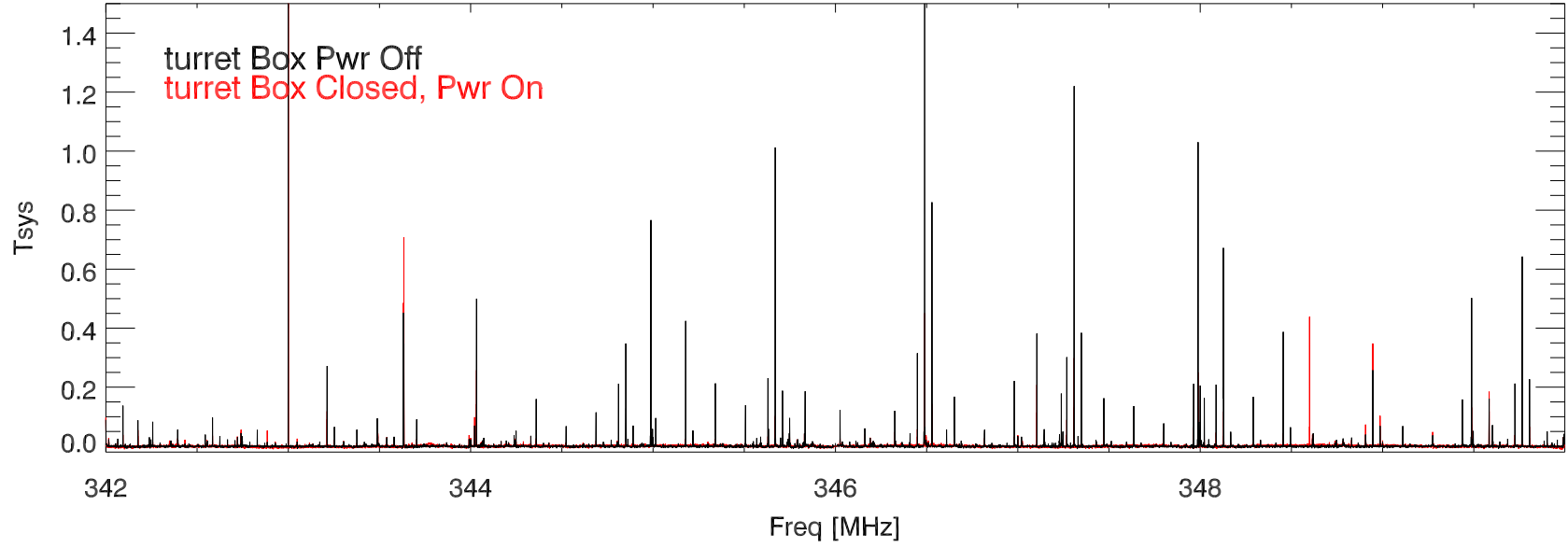
28jan16 327 rcvr. turBox on, off bm6
