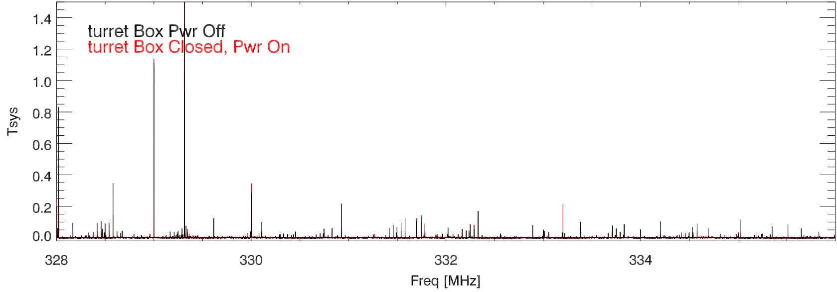
28jan16 327 rcvr. turBox on, off bm4
