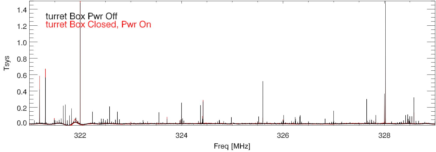
28jan16 327 rcvr. turBox on, off bm3
