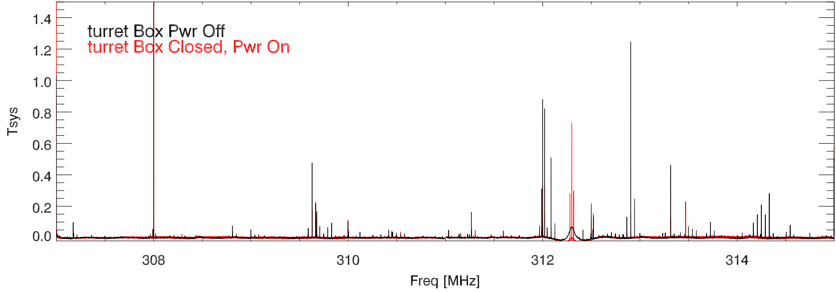
28jan16 327 rcvr. turBox on, off bm1
