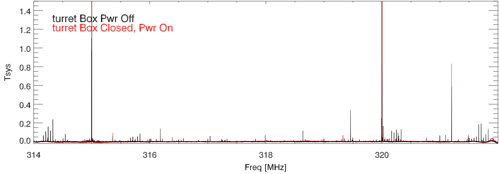
28jan16 327 rcvr. turBox on, off bm2
