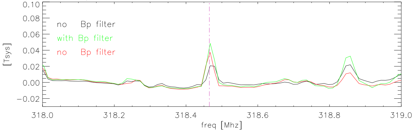
10jan06 327 rcvr. polB green trace bp filter. 318.465 birdie gone
