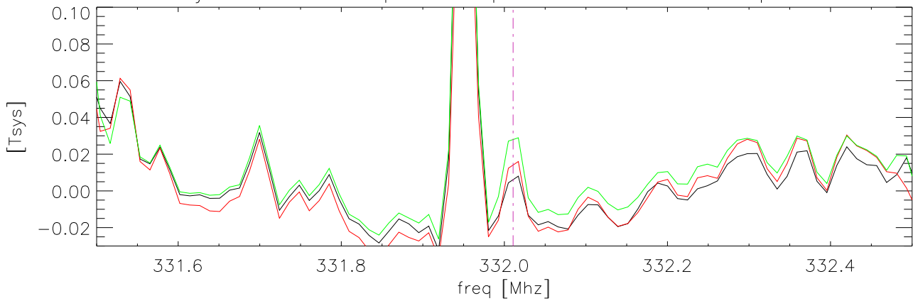
10jan06 327 rcvr. polB green trace bp filter. 332.011 birdie gone
