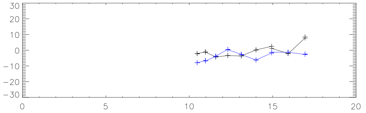
B2209+080 az,za error vs za
