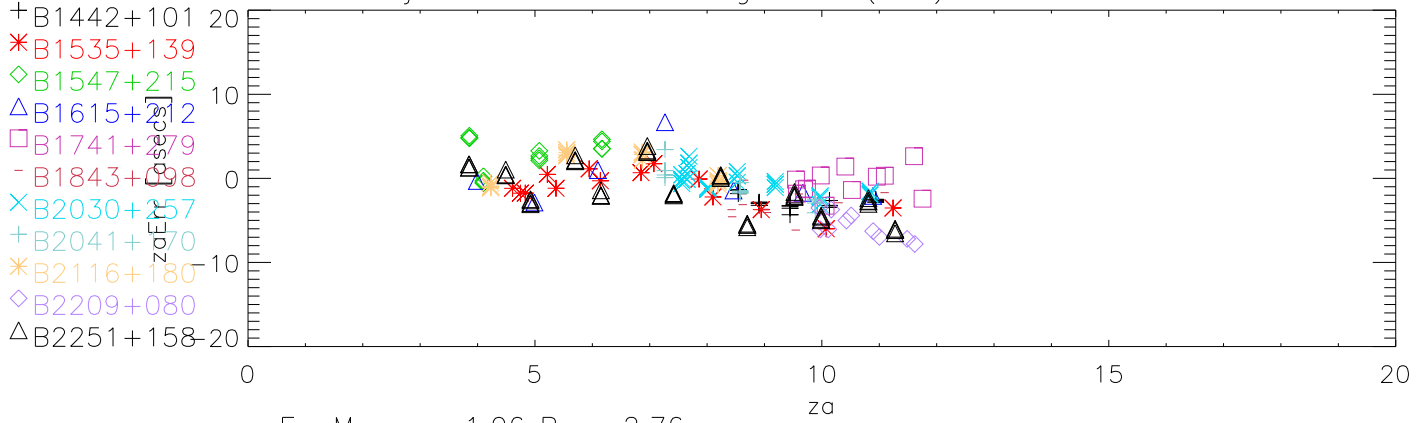
09jun10 after correcting za sin(3az) term za error vs za
