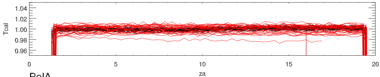
16apr11 a2130 alfaCalDeflection vs za beam0
