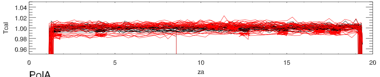
14nov11 a2130 alfaCalDeflection vs za beam0
