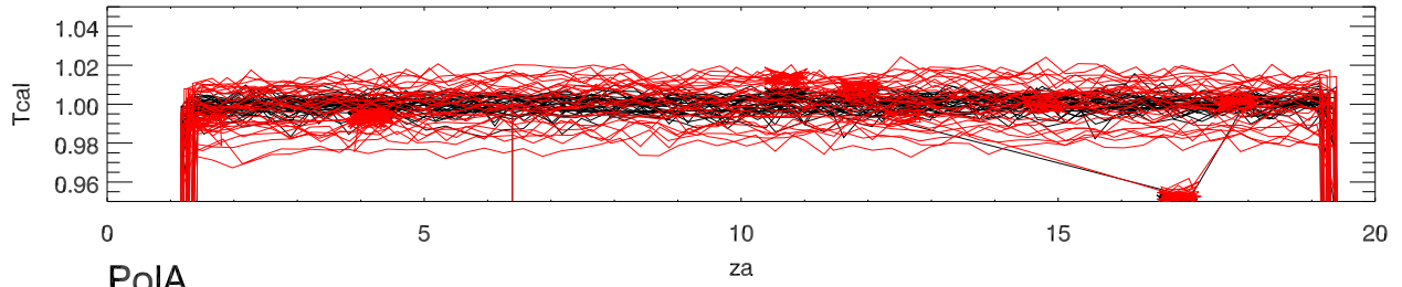
01nov11 a2130 alfaCalDeflection vs za beam0
