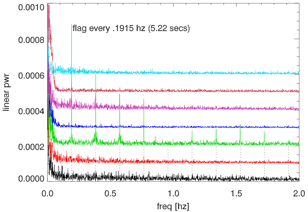
PoIB
