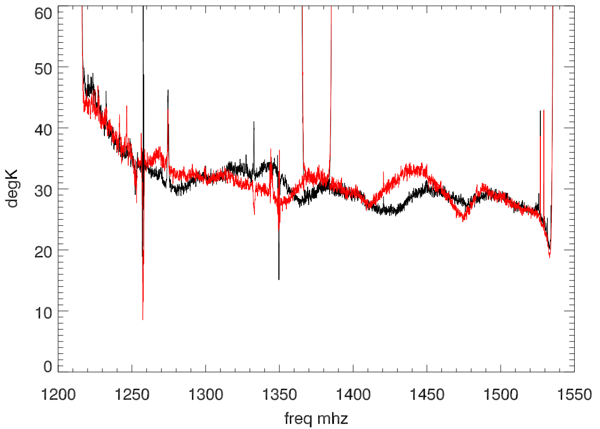
06jan14, alfa bandpass in degK
