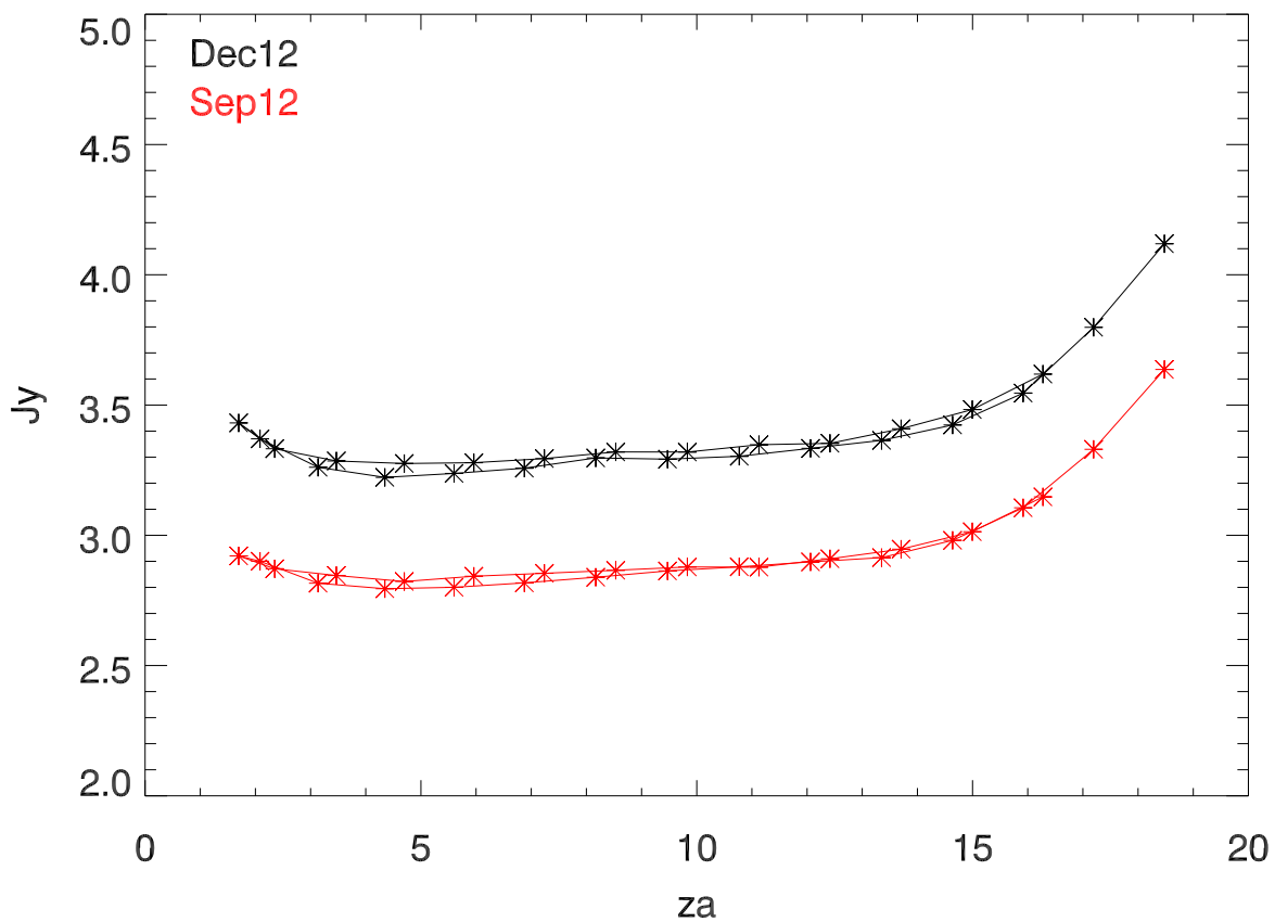
lbw sefd 3C138 sep12,dec12
