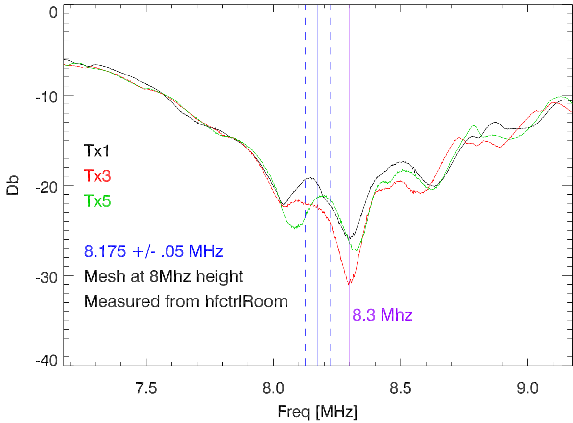
02aug2018 S11 vs Freq 8Mhz radial dipoles: 1,3,5
