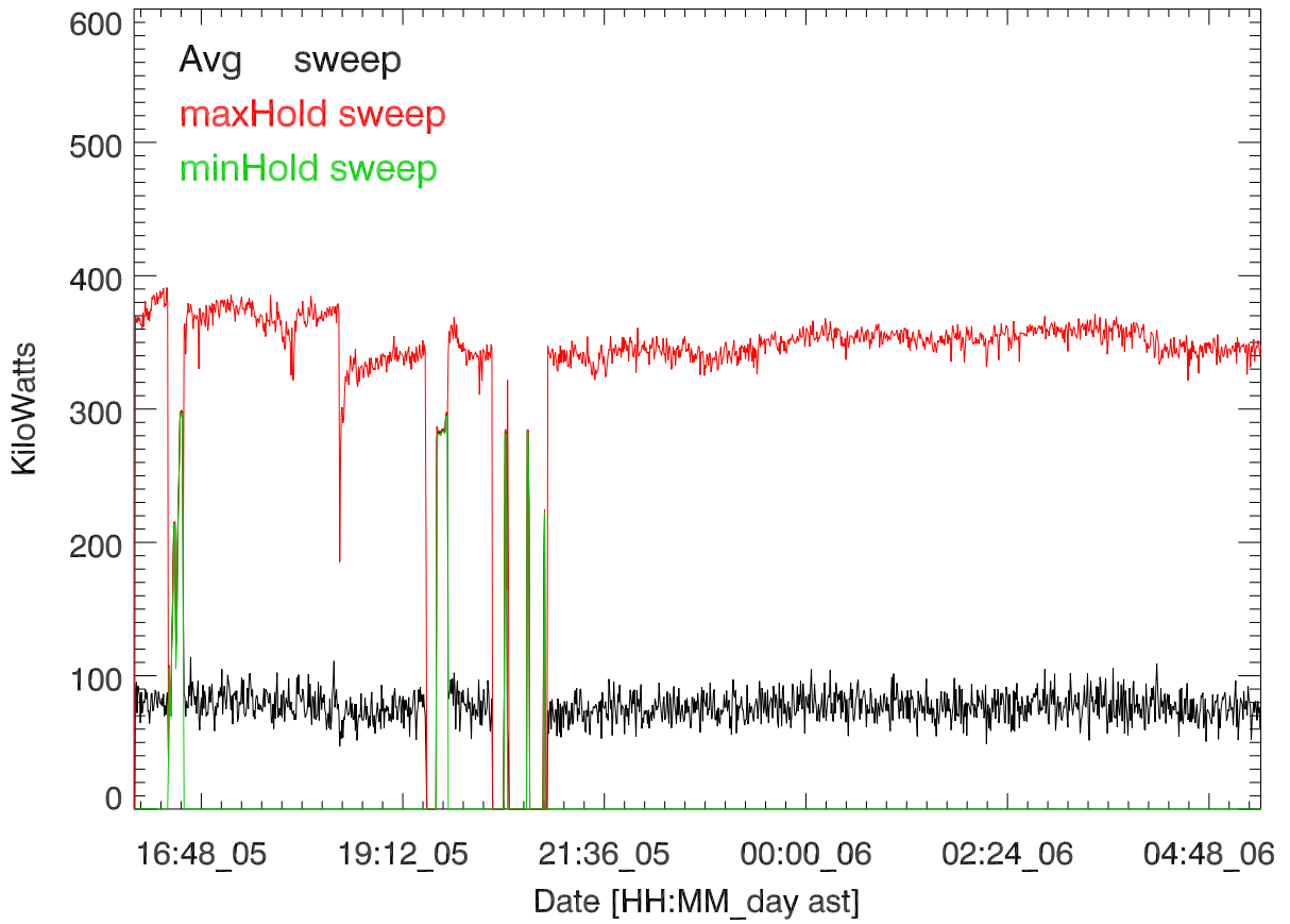
TxPwrTot. 05oct16:T2915. Salih Bostan 8 MHz
