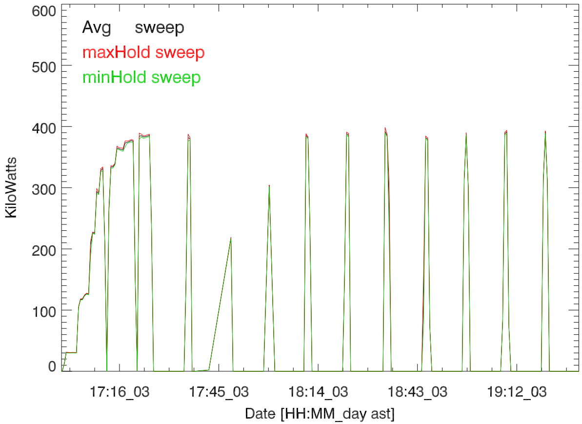
TxPwrTot. 03nov16:H1111. Frank & Herb. 5 MHz
