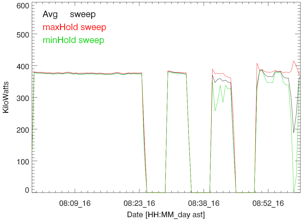
TxPwrTot. 16mar17:H3156. Paul Bernhardt epop5 MHz
