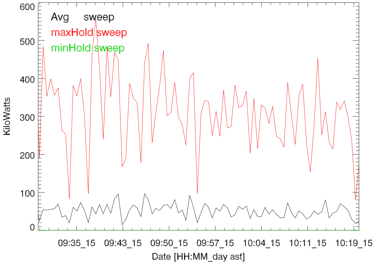
TxPwrTot. 15mar17:t2915 Salih Boston. 5 MHz
