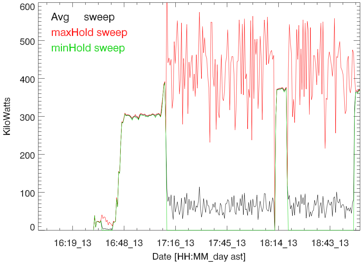
TxPwrTot. 13mar17:T2915. Salih Boston 8 MHz
