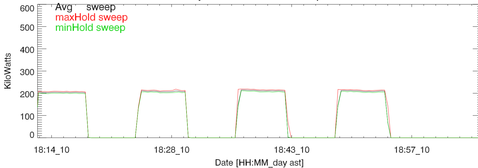
TxPwrTot. 10jun19:H3195 vladimir exp10.11 5 MHz
