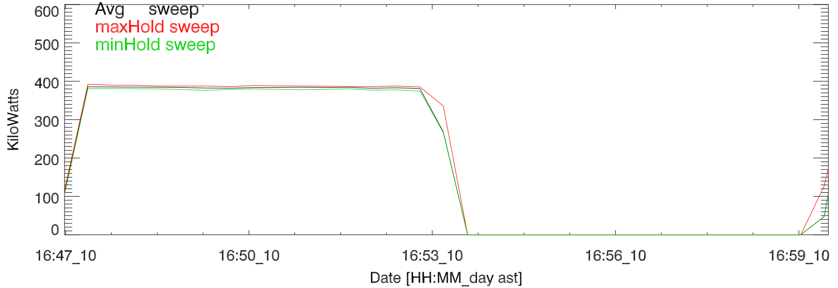
TxPwrTot. 10jun19:H3195 vladimir exp10.08 5 MHz
