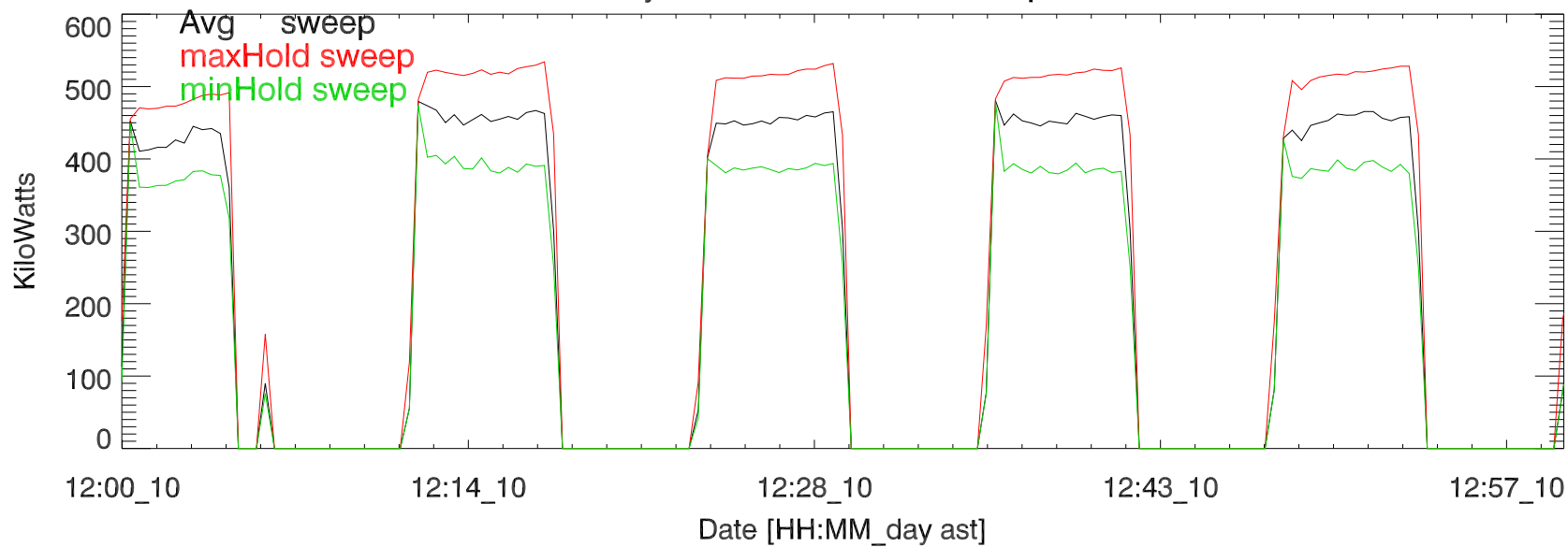
TxPwrTot. 10jun19:H3195 vladimir exp10.04 5 MHz
