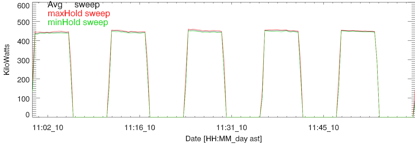
TxPwrTot. 10jun19:H3195 vladimir exp10.03 5 MHz
