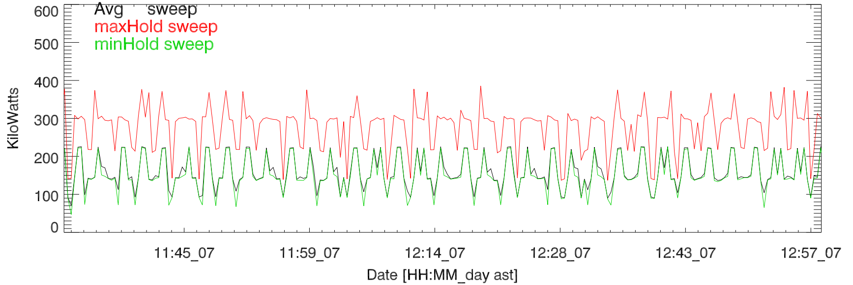
TxPwrTot. 07nov18:H3251 5 MHz
