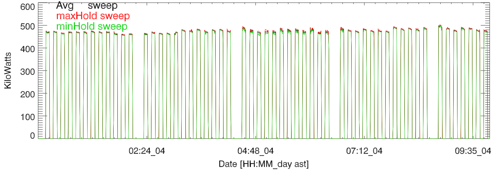
TxPwrTot. 04nov18:H3108 5 MHz
