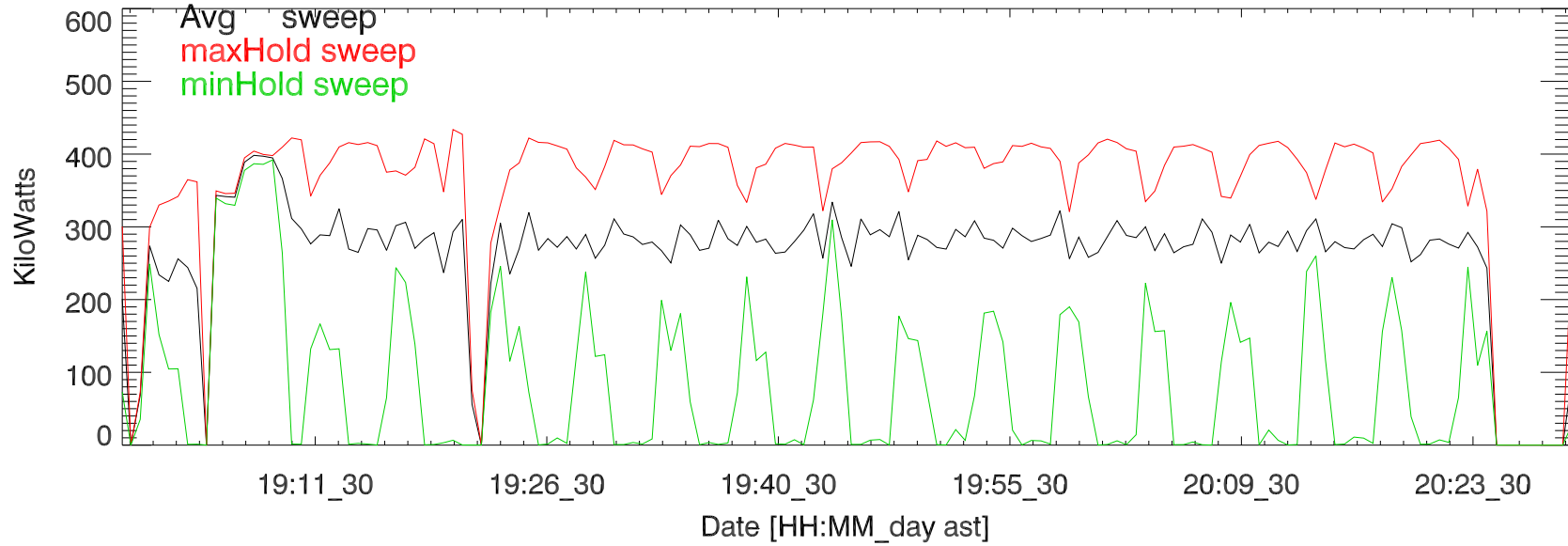
TxPwrTot. 30jul17: Hunter 5 MHz
