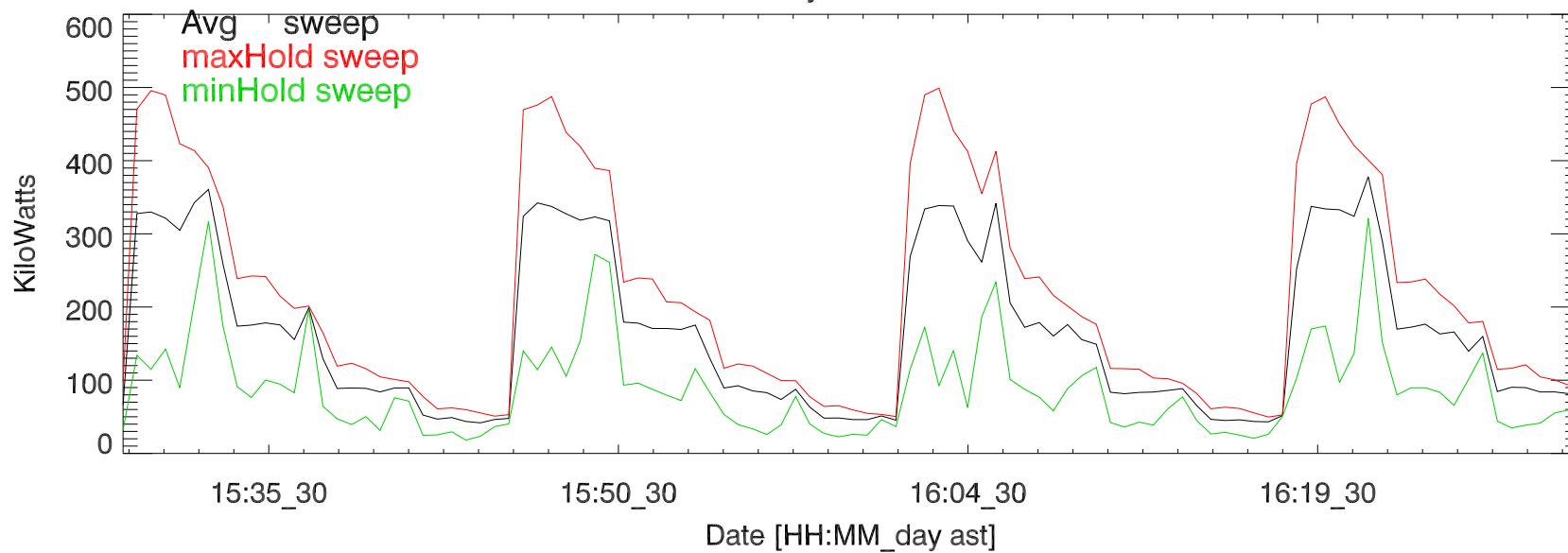
TxPwrTot. 30jul17: Jamie 5 MHz
