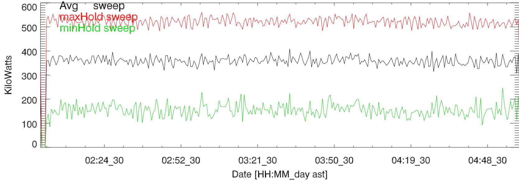
TxPwrTot. 30jul17: Jackson 5 MHz
