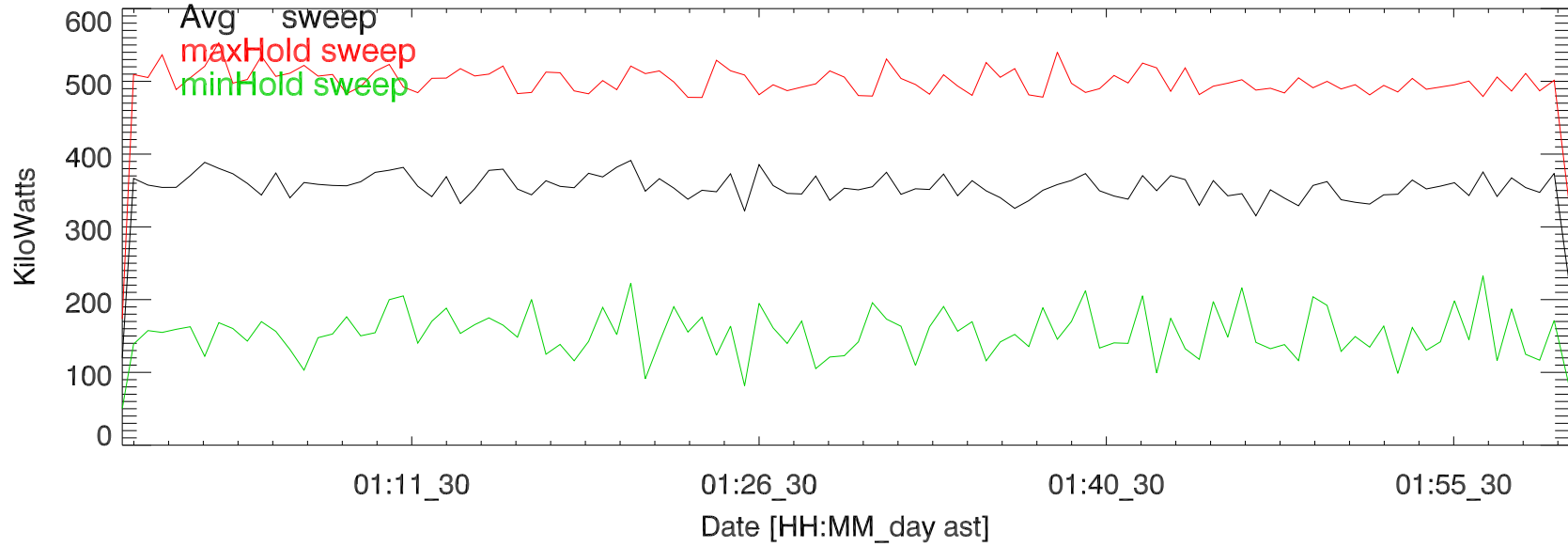
TxPwrTot. 30jul17: Quincy 5 MHz
