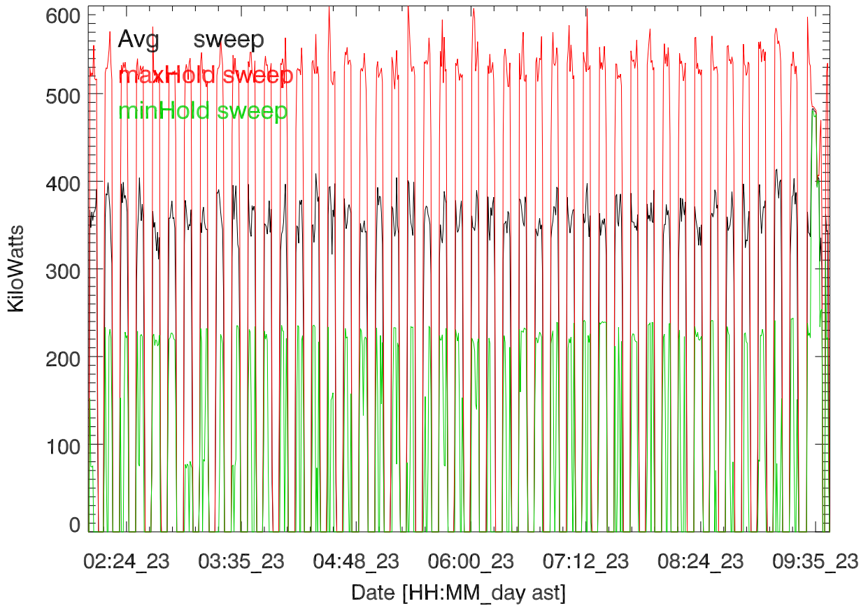
TxPwrTot. 23may17:H3171. Eliana Nossa. 5 MHz
