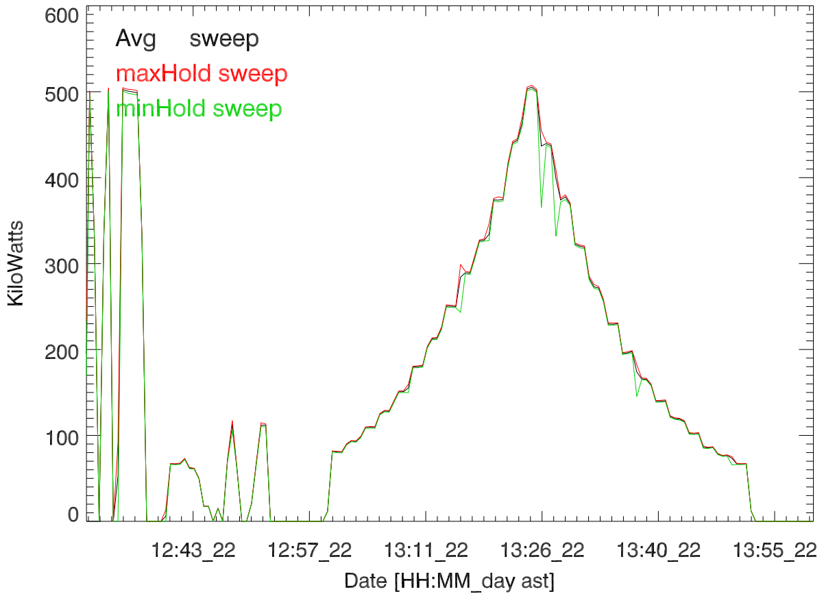
TxPwrTot. 22may17:H3171. Eliana Nossa. 5 MHz
