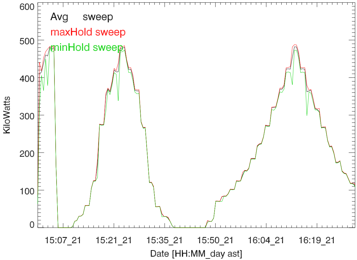
TxPwrTot. 21may17:H3171. Eliana Nossa. 8 MHz
