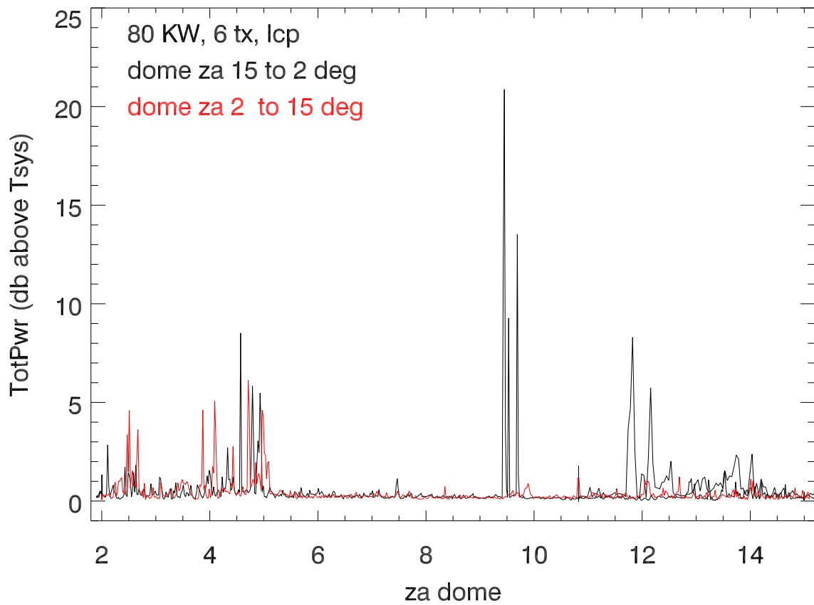
02nov15 hfOn: dome total power vs za (az=348)
