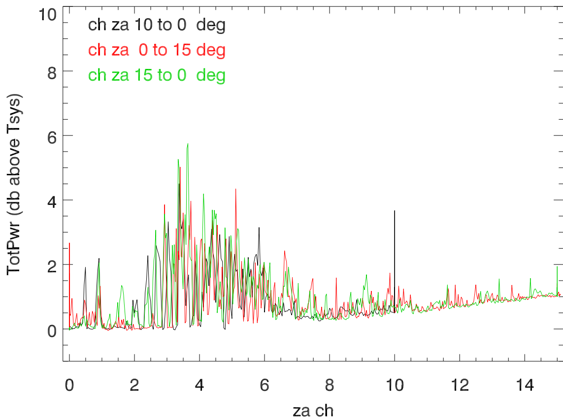
ch total power vs za (azGr=348)
