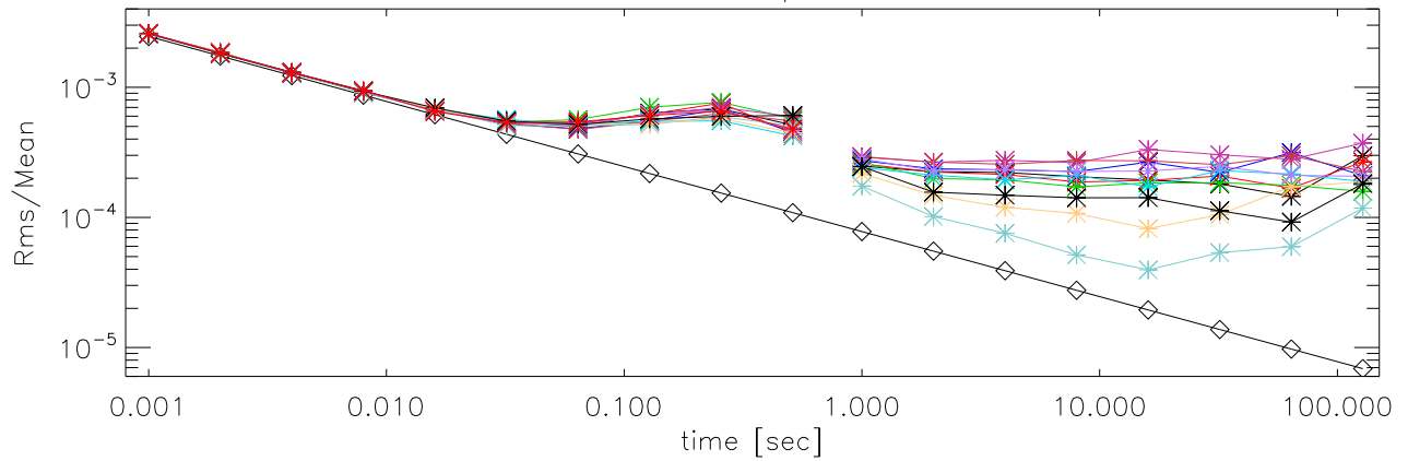
hiBand polB
