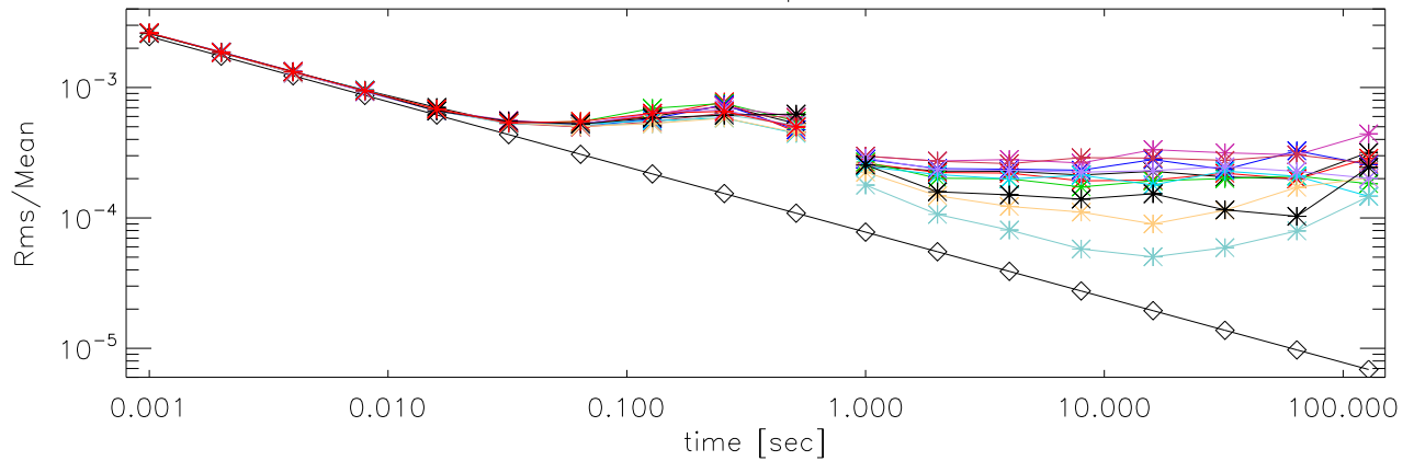
hiBand polB
