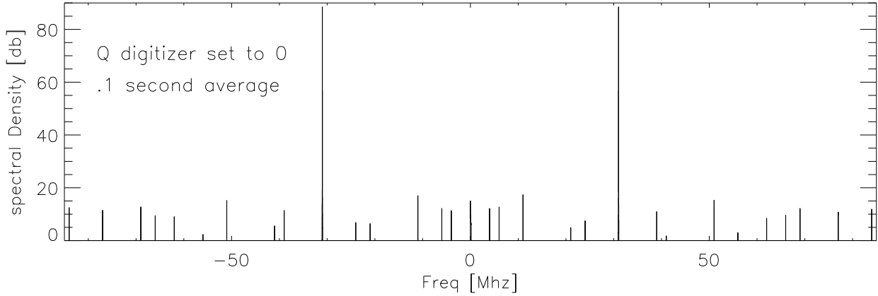
Pk A/D=414 cnts (pshift=0x1ff5)
