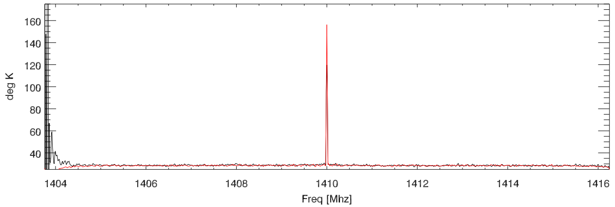
PoIB bw=12.5Mhz
