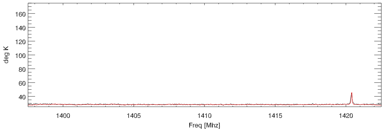
PoIB bw=12.5Mhz
