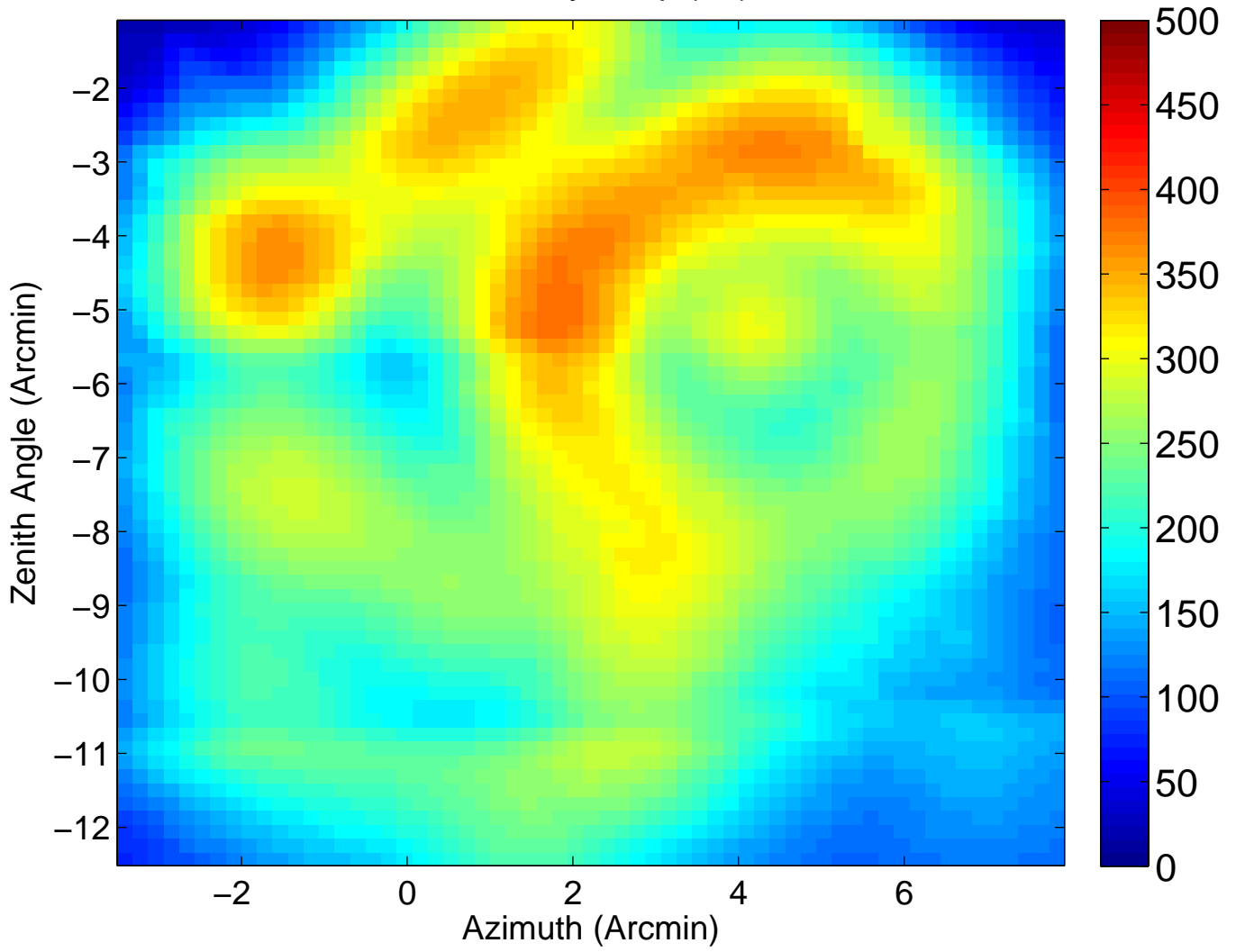
A6 Ae/Tsys Map (A6)
