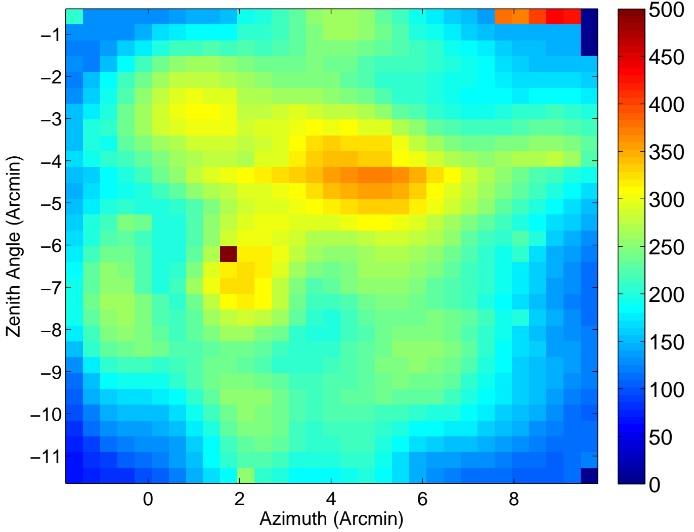
A4 Ae/Tsys Map ( z = 7.454 cm)
