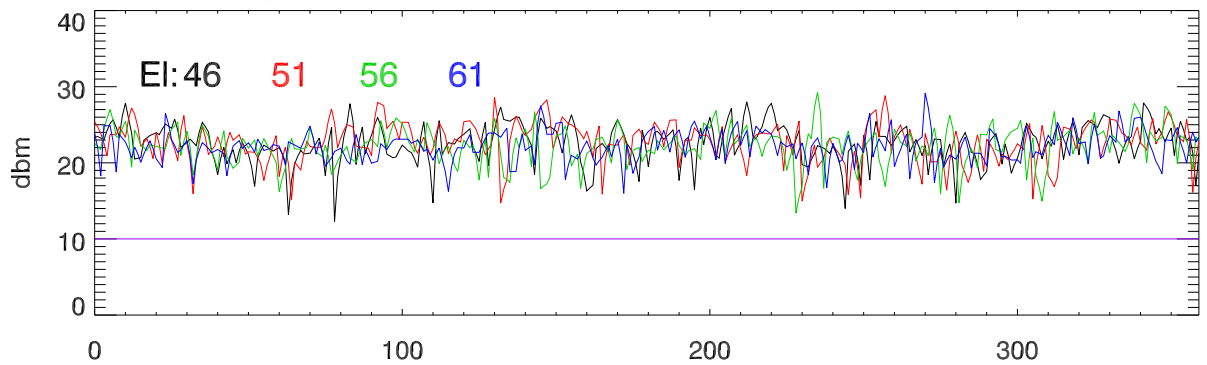
17may23 azswings total pwr (2-12GHz @ FoTxInpNoPads) vs az
