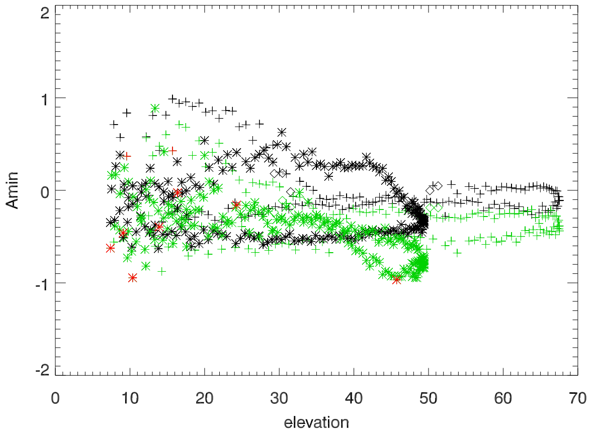
Pointing error. az,el error vs el
