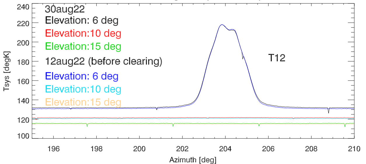
220830: azswing blowups. cfr 8219 polA
