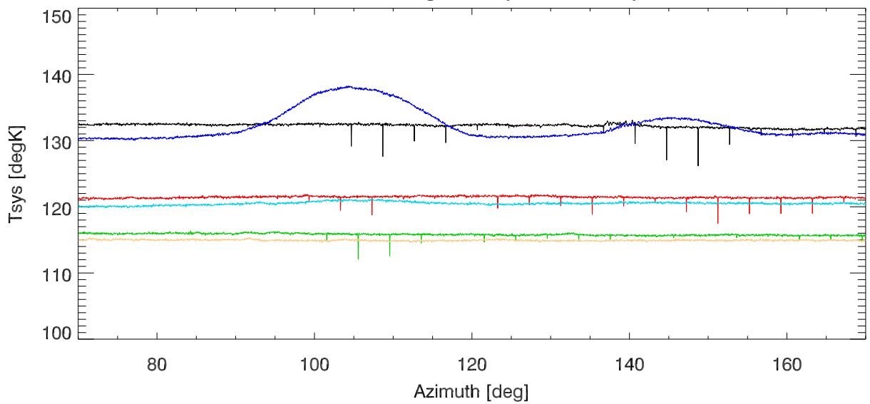
220830: azswing blowups. cfr 8219 polA
